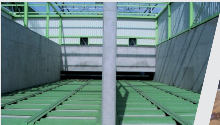
Silo avec convoyeurs à raclettes ZENO pour centrale biomasse
